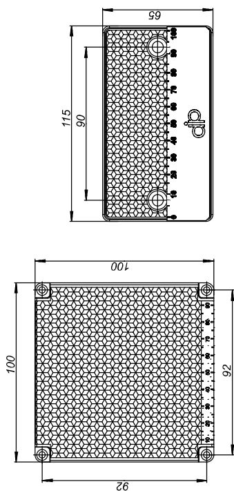
Рефлектор-отражатель ДПРМ.203625.004 (тип СМ) (см. табл. 1)
