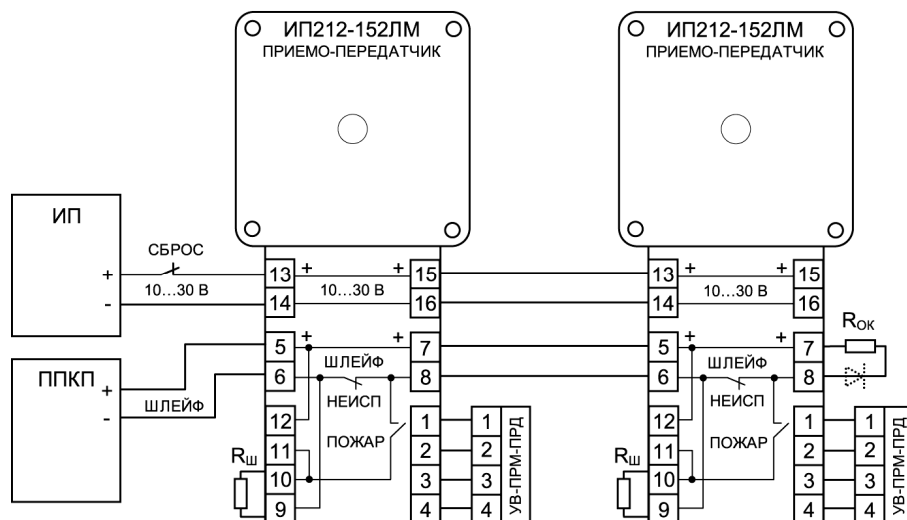
Рисунок 8 (Схема 2-2)
