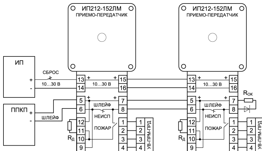
Рисунок 7 (Схема 2-1)
