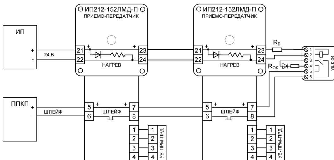
Рисунок 5 (схема 7-2)
