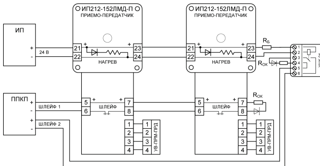
Рисунок 4 (Схема 7-1)
